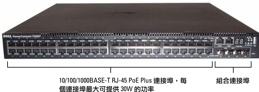
圖 1-5. PowerConnect 7048P，具有 48 個 10/100/1000BASE-T PoE Plus 連接埠
